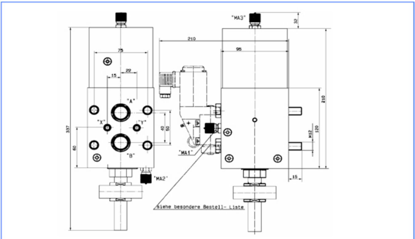
* Maßbeispiel Senk-Brems-Sperrventil DN 16, 320 bar
